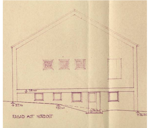
Figur 11 Fasad nordöst
