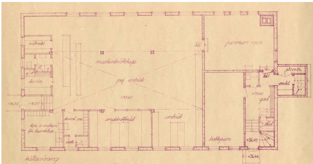
Figur 15 Källarvåning med andelstvätter
