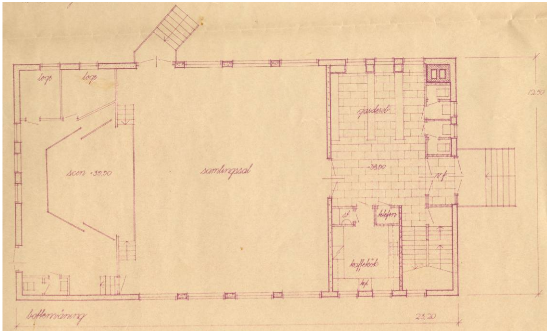
Figur 14 Planritning samlingslokal och kök
